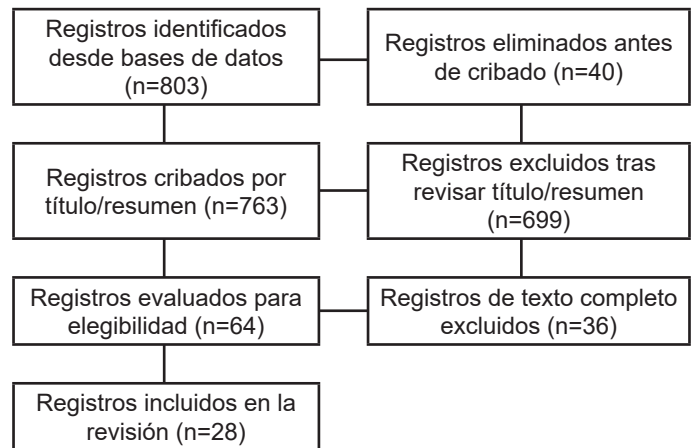
Figura 1. Diagrama de flujo PRISMA para explicar el proceso de selección de los artículos a través de las bases de datos.
